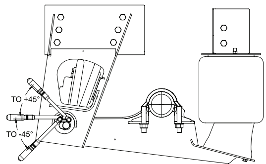
QUIK-ALIGN®
